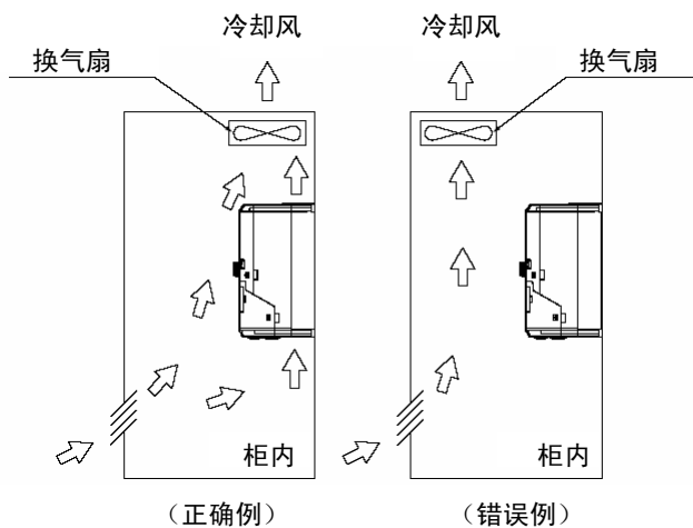
图 3-4 柜内换气扇的安装位置
