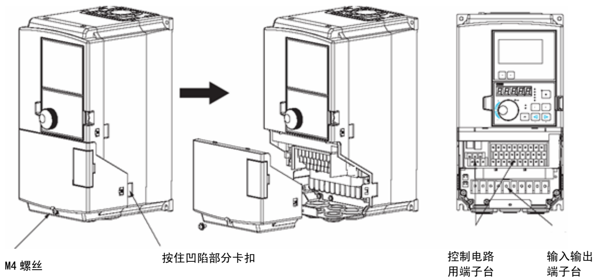
图 3-5 前盖板（下）拆卸
