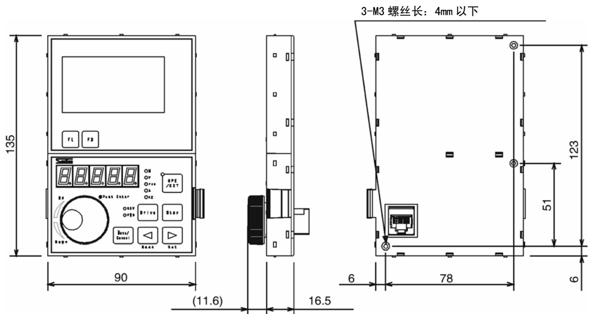
(1) 操作面板
