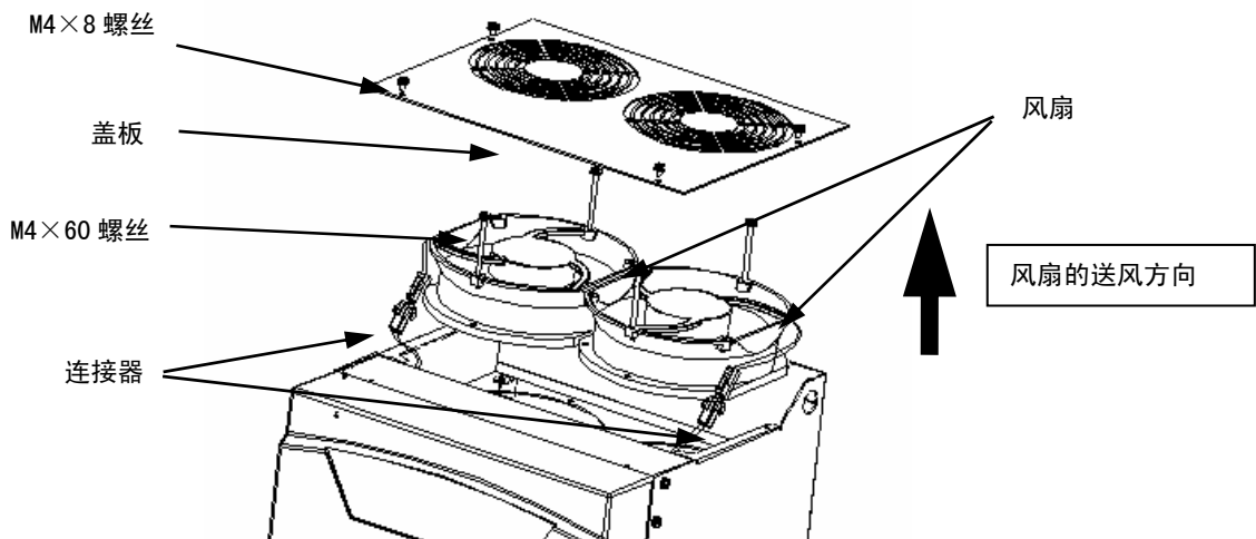
图 10-5 风扇的更换步骤 (SVC06-0550~0750)
